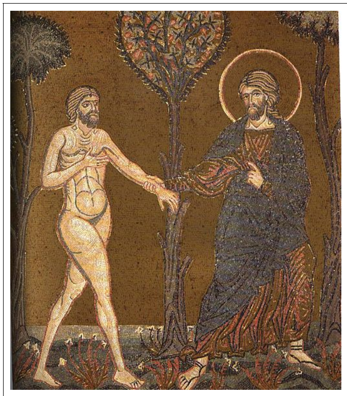
Adam komt tot Eden.
